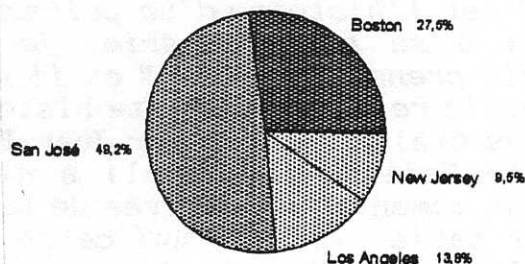
% DE PUNITIONS PAR ÉQUIPE PAR RAPPORT AUX AUTRES CLUBS
