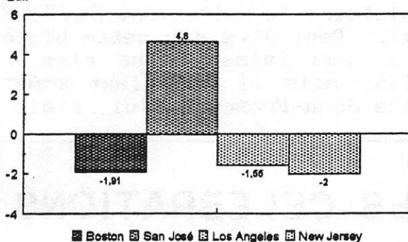
MOYENNE DE LA DIFFÉRENCE BP-BC PAR MATCH
